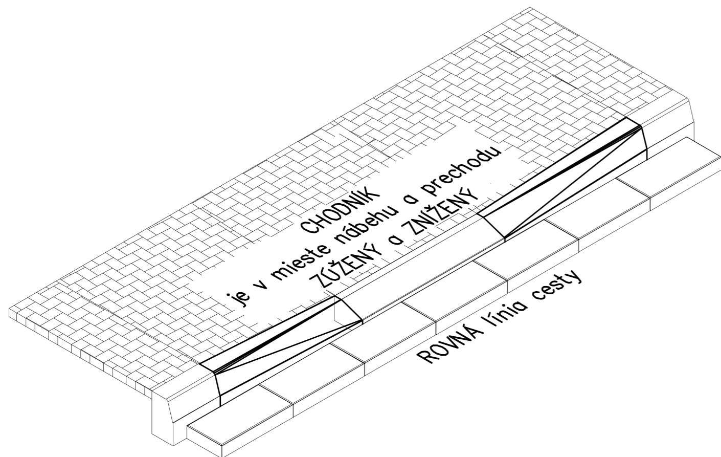
Pohľad čelný
